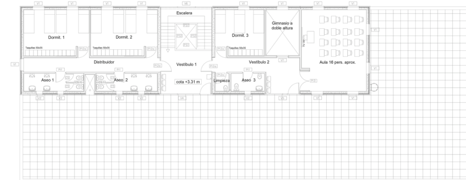
Planta Primera
