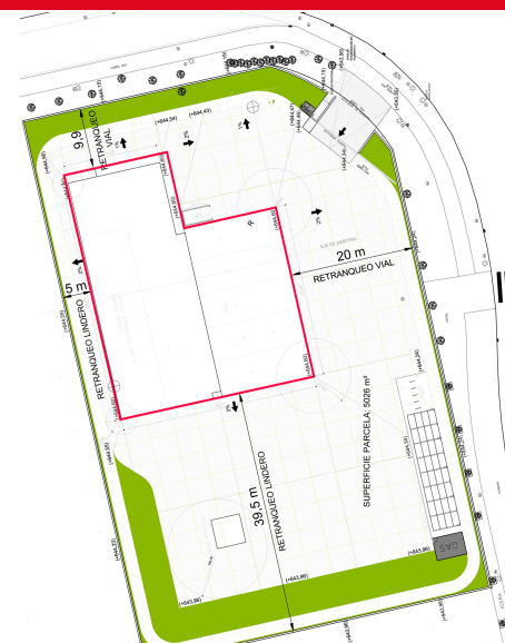
Planta General
